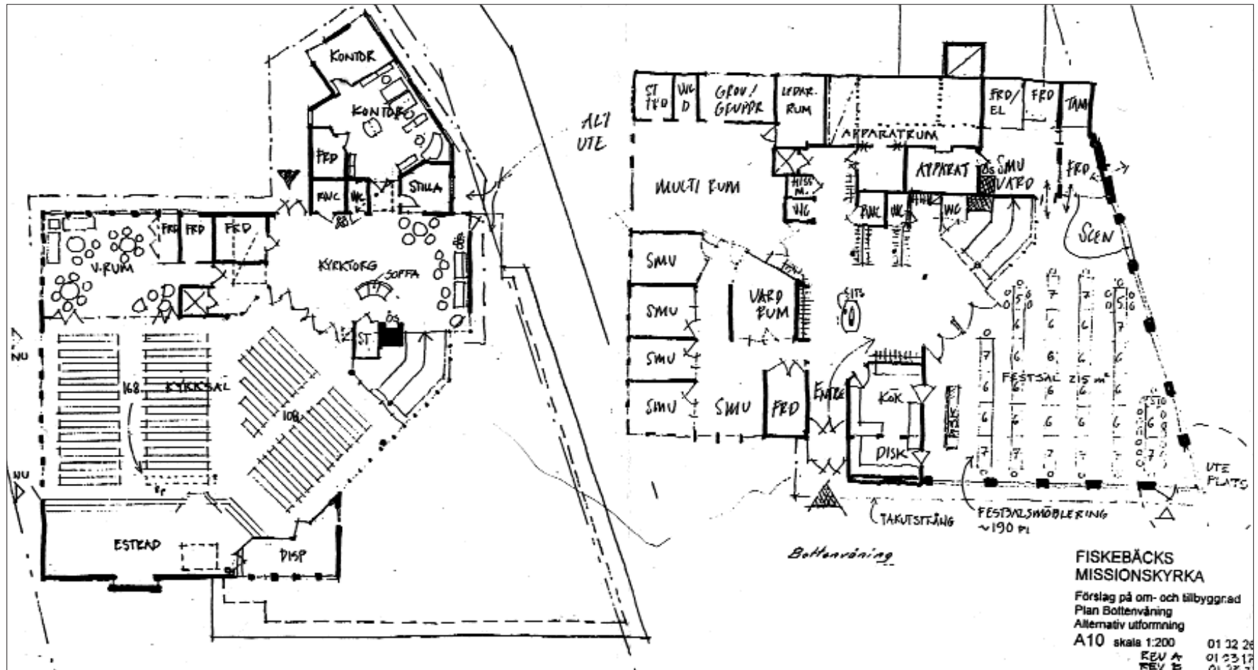
Så här är förslaget till om- och tillbyggnad av Fiskebäcks Missionskyrka. Till vänster syns det övre planet, till höger det nedre. Sammanlagt handlar det om 475 nya kvadratmeter. Vill du se ritningarna i större format är du välkommen till kyrkan. Ritning: LINDFORS ARKITEKTKONTOR AB
